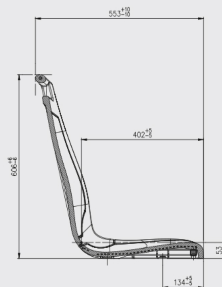
Sez. A-A
